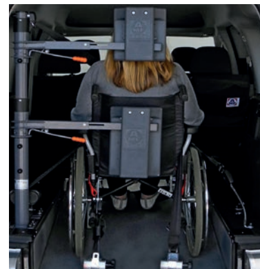
Das Fahrzeug kann mit der Kopf- und Rückenstütze Future Safe ausgestattet werden.
